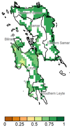
NDVI
