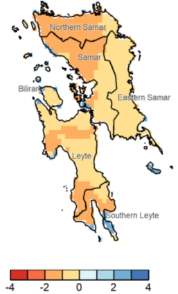
SPEI3 (Mar-Apr-May)
